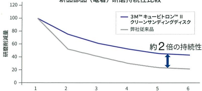
新品部品（電着）研磨持続性比較
