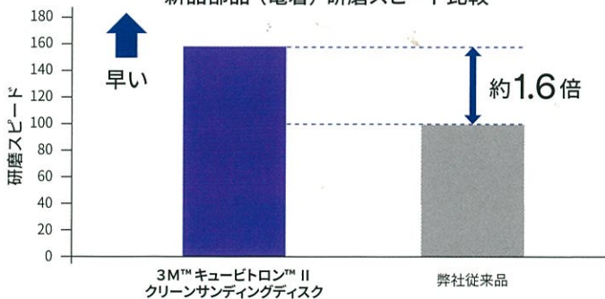
新品部品（電着）研磨スピード比較
