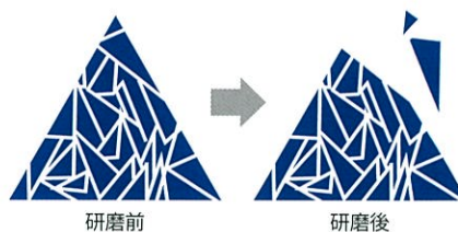
精密成型砥粒 研磨砥粒の研磨前、後のイメージ図
